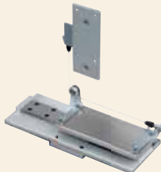
90度での剥離
