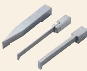
QFP リードフック/チップせん断治具
