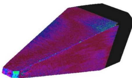
ボンディングツール先端部の差分解析(未使用品と使用済み品との比較評価)
