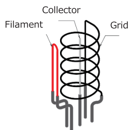
SH200測定子内部
