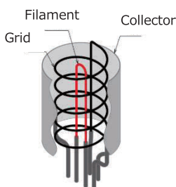
ST200測定子内部
